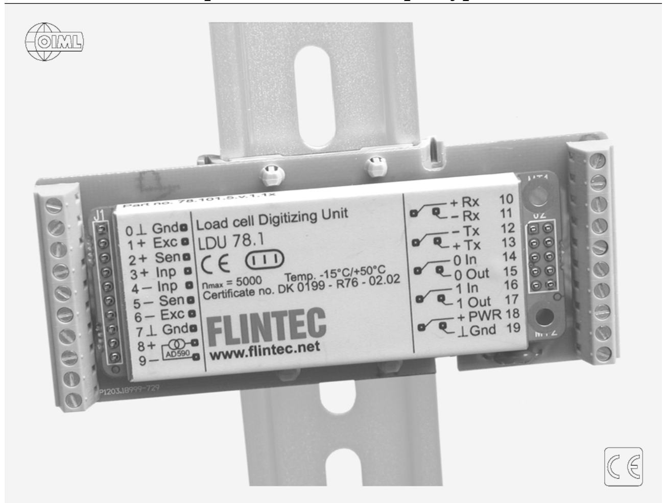
LDU 78.1 fixé sur la carte adaptateur optionne Ile UA 77.1
